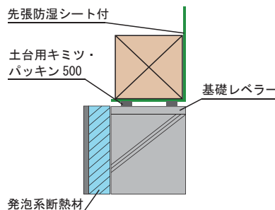
土台部分の施工
