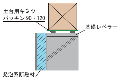
土台用キミツ・パッキン 90・120 の使用図
