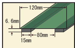
土台用キミツパッキン 120
