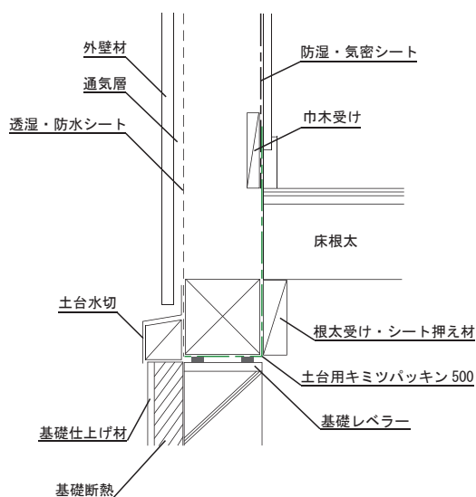
土台部分の施工
