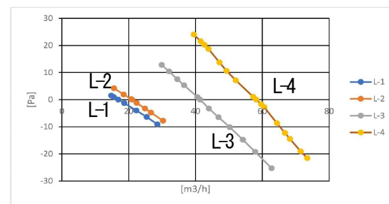
PQ曲線図 給気
