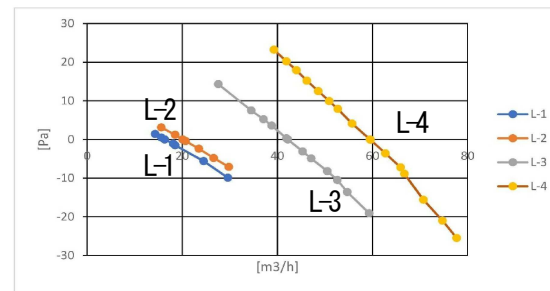
PQ曲線図 排気
