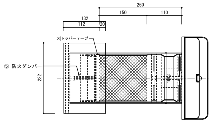
機器平面図
