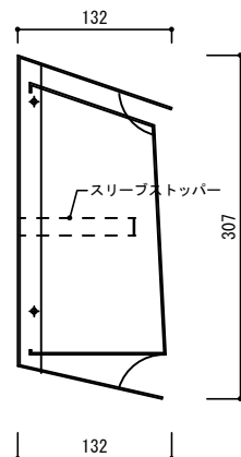
耐風圧アウターフード 断面図 【コンパクトXL】
