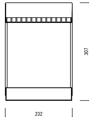
耐風圧アウターフード 正面図 【コンパクトXL】
