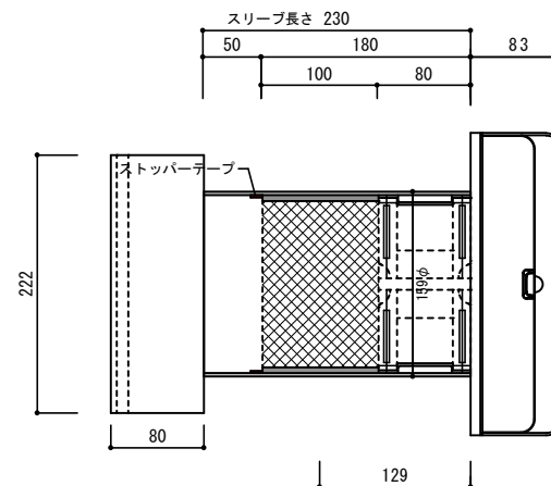
機器平面図
