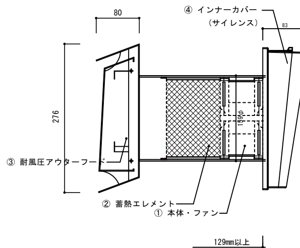
機器側面図
