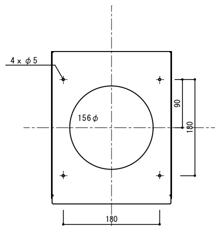
ベースプレート
