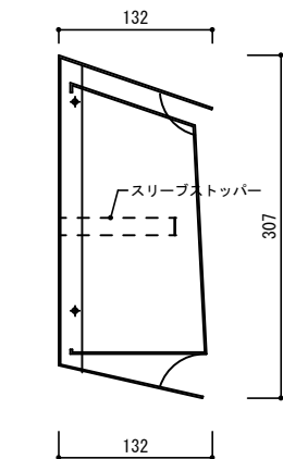
耐風圧アウターフード 断面図 【コンパクトXL】
