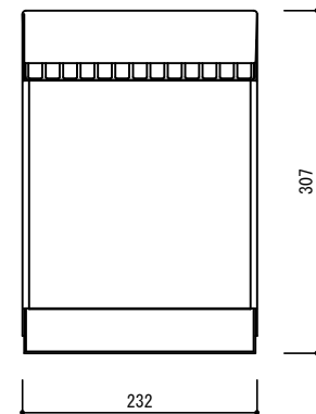
耐風圧アウターフード 正面図 【コンパクトXL】 機器側面図
