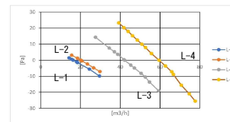
PQ曲線図 排気
