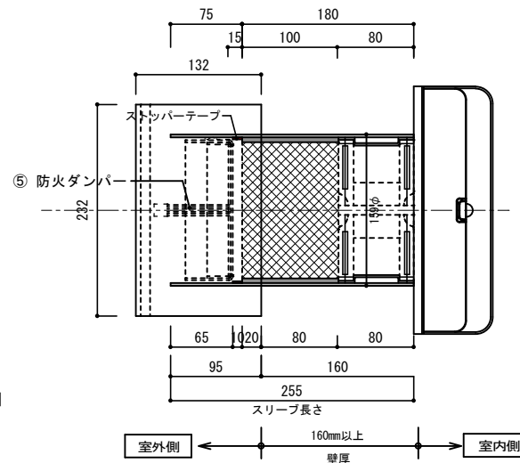
機器平面図 耐風圧アウターフード背面図 【コンパクトXL】
