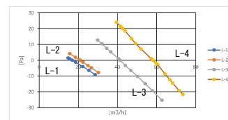
PQ曲線図 給気
