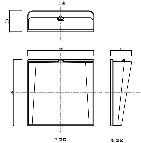
正面図
