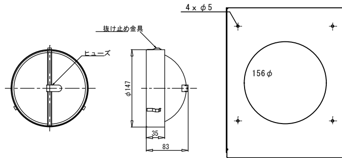
防火ダンパー
