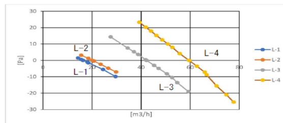
PQ曲線図 排気
