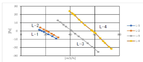
PQ曲線図 給気
