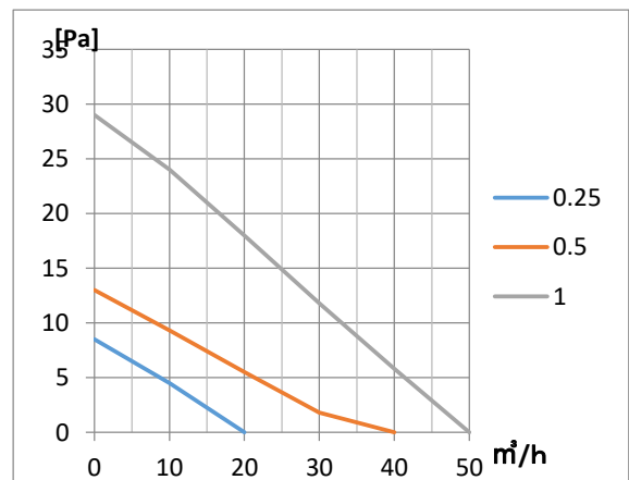
PQ曲線図
