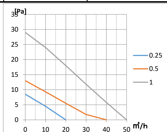
PQ曲線図
